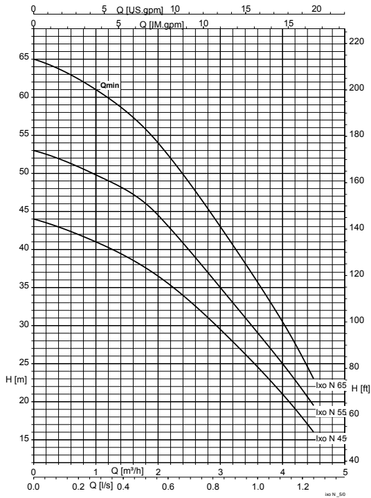
Ixo N 45/55/65; n = 2900 min -1
